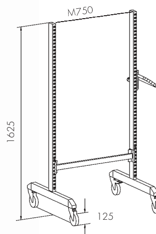
Rama wózka Basic
